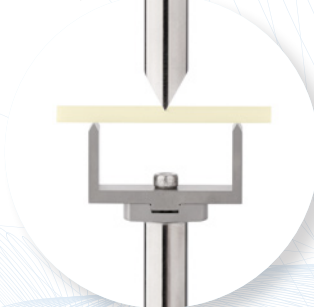
DMA 三点弯曲
