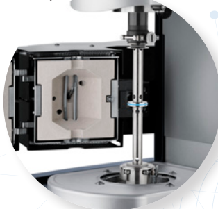
强制对流炉 (FCO)
